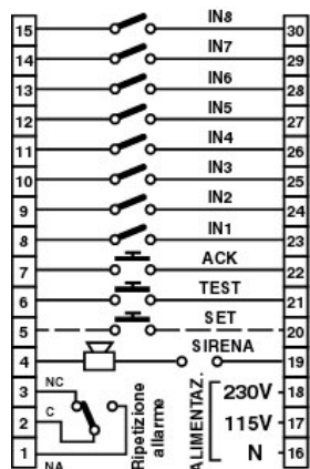
Morsettiera
